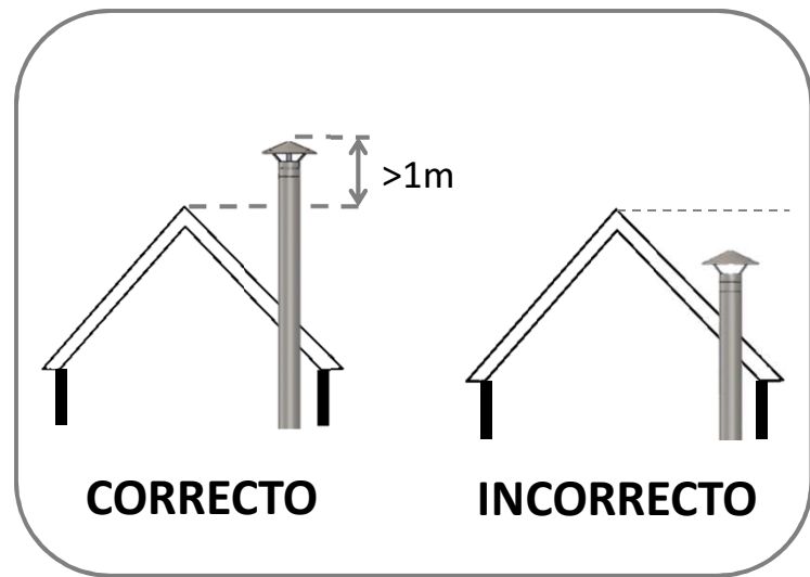
1ª Caso.- Sombrerete por debajo de la línea de cumbrera.
