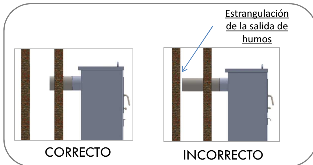
4º Caso.- Estrangulación del tubo de la salida de humos.
