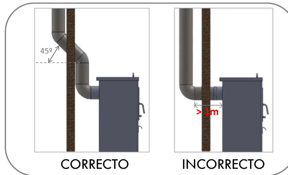
5ª Caso.- Tubo macizado debido a un tramo horizontal (acumulación de hollín).
