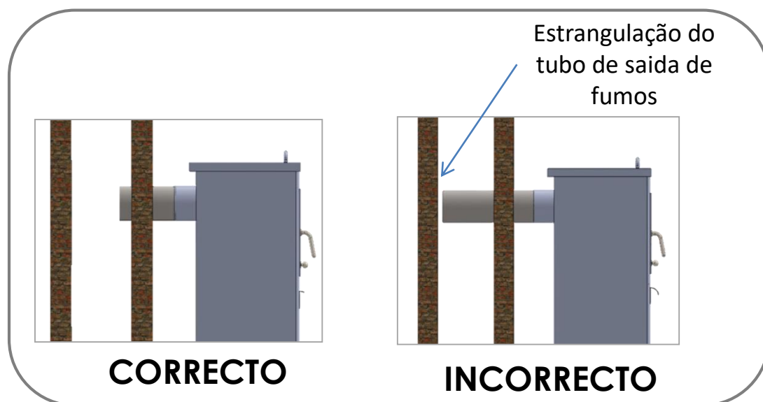
4 o Caso.- Estrangulação do tubo de saída de fumos
