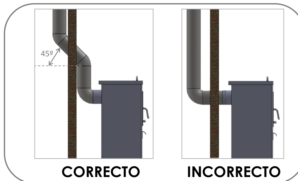
5 o Caso.- Estragulamento tubo devido a uma seção horizontal (acumulação de fuligem).
