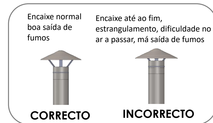
3 er Caso.- Chapeu enfiado até ao final
