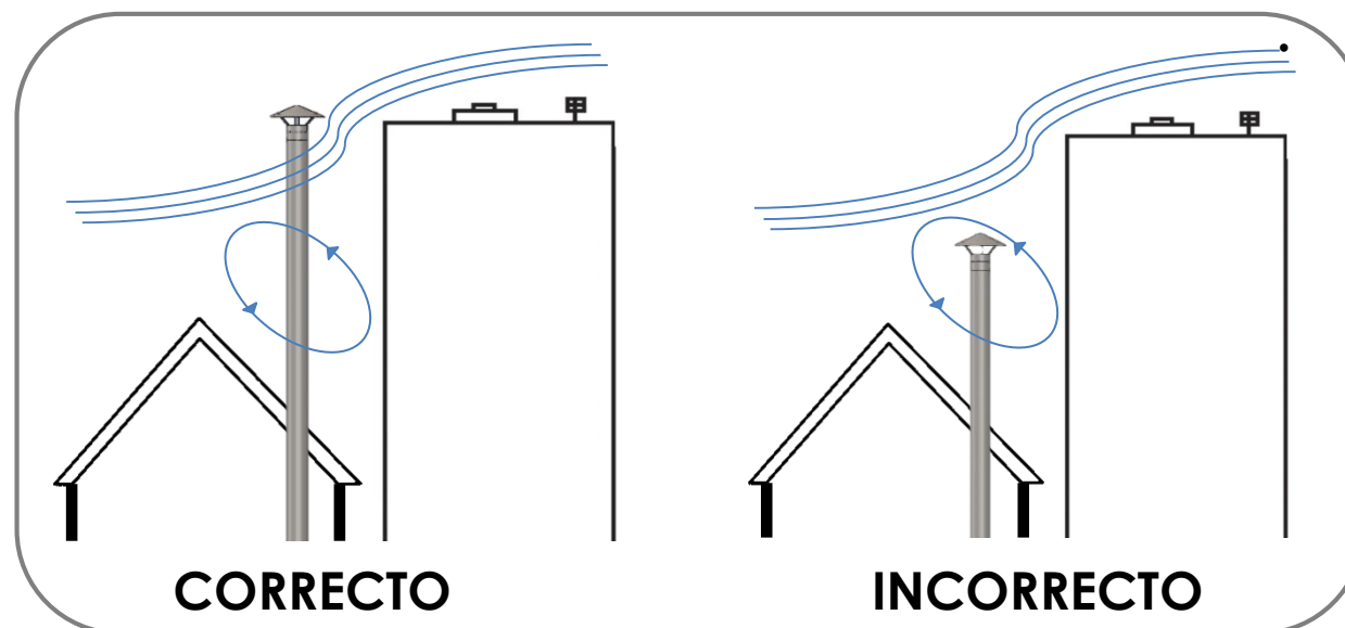
2 o Caso.- Chapeu por cima da linha da cumeeada mas próximo de um edificio mais alto
