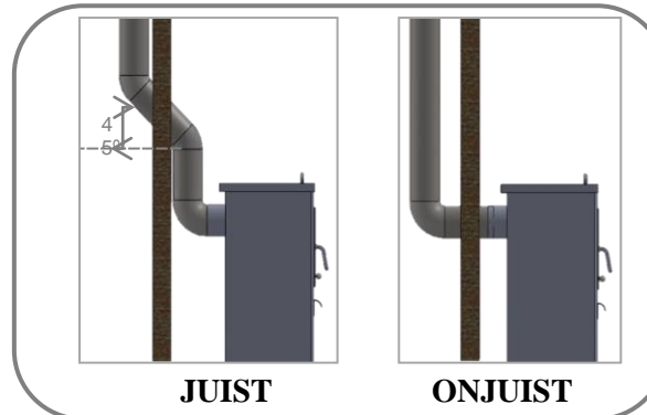
5e Geval. - Buis verstopt door een horizontale bocht (ophoping van roet).
