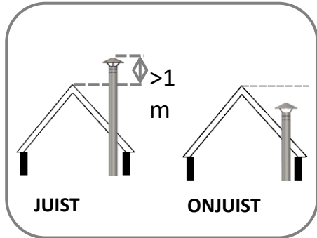
1e Geval. - Schoorsteenkap onder de lijn van de nok.
