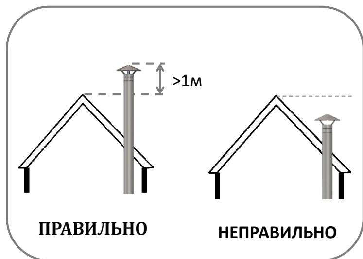
Ситуация 1. - Дымоходная труба находится ниже линии хребта крыши
